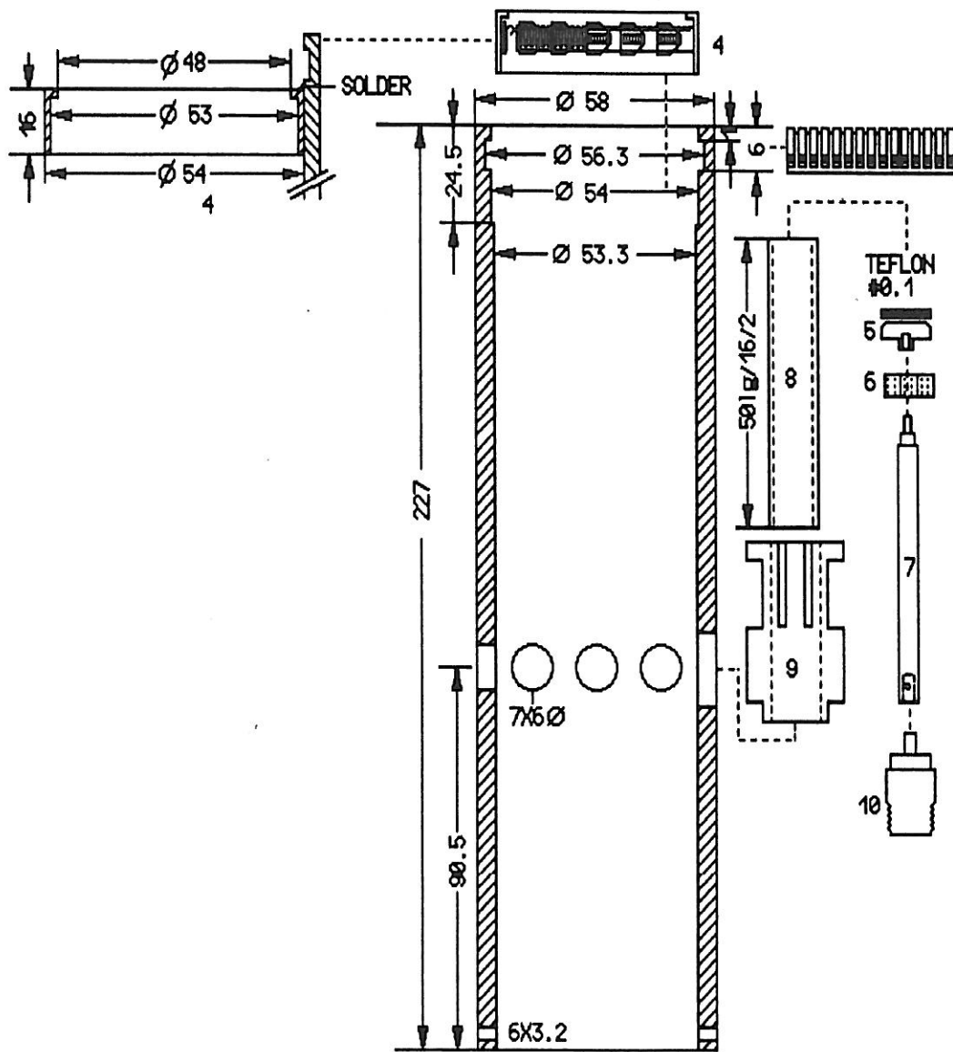
Screen en toebehoor DL9EBL cavity 1296 MHz
