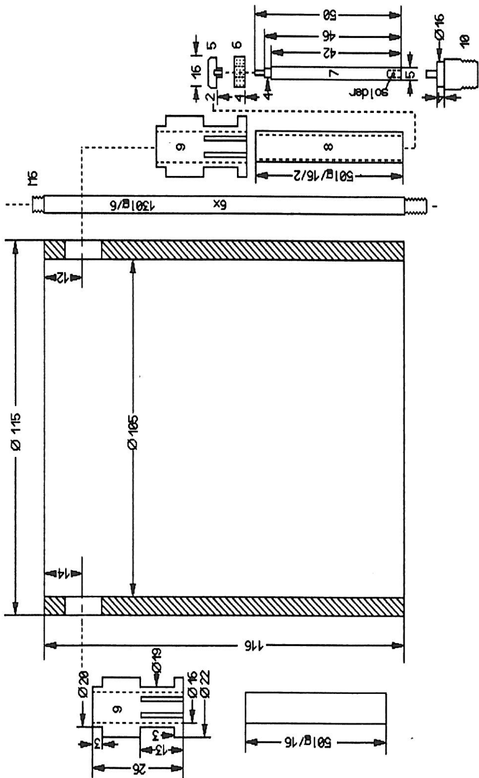
Anode deel DL9EBL cavity 1296 MHz
