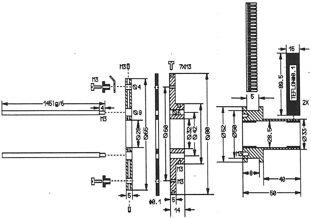
Kathode deel DL9EBL cavity 1296 MHz
